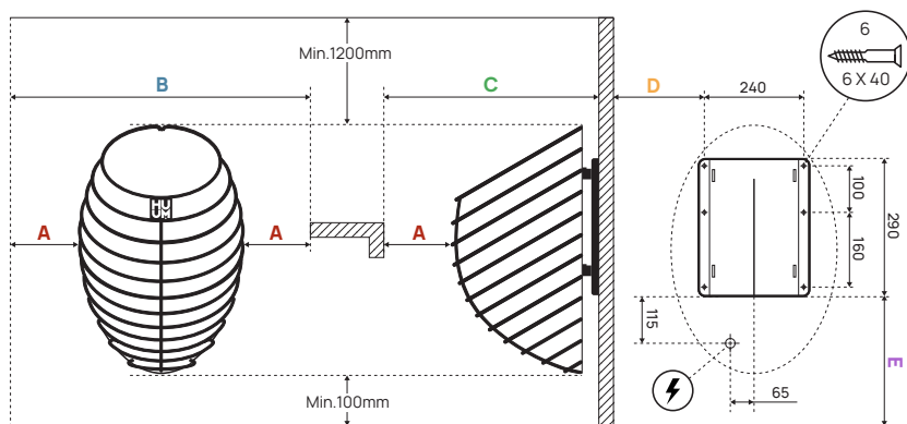
Postava 1. Instalace ohříváče
